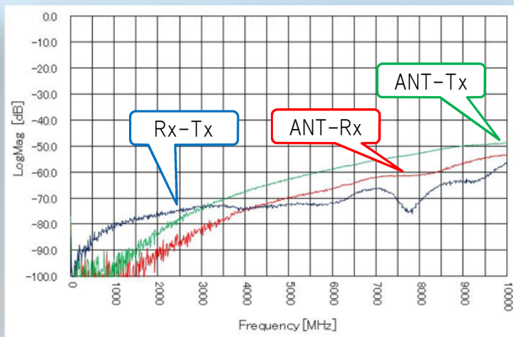
各Port間のアイソレーション特性
