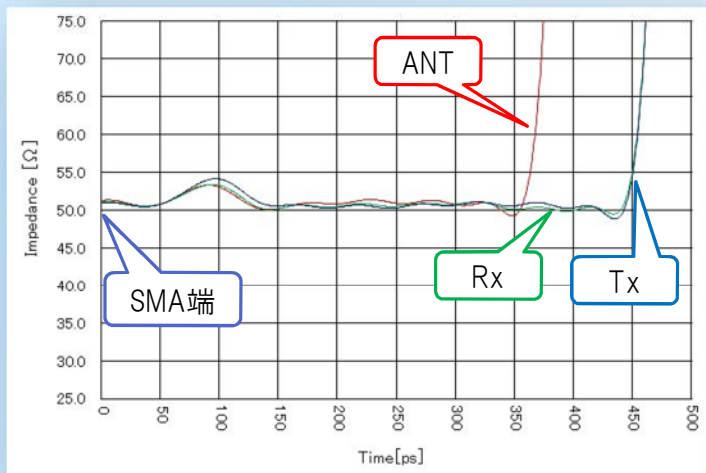
各Portのインピーダンス特性
