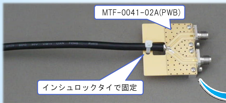
モード変換(Sdc11): 基板+SMALレセプタクル
