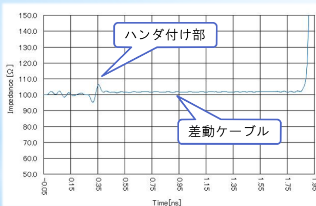
Impedance: 差動ケーブル測定 (Tr=35[ps])
