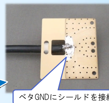
モード変換(Sdc11): 基板+SMALレセプタクル
