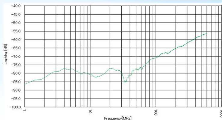
モード変換(Sdc11): 基板+SMALレセプタクル
