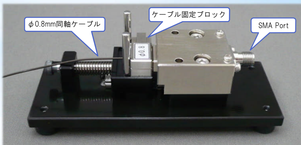
同軸ケーブルのセット
