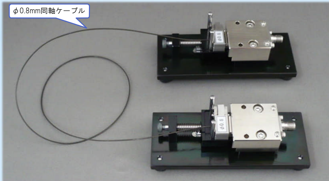
測定セットアップ
